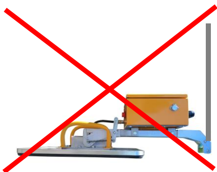
Рисунок 6.3.1 Позиционирование захвата при подъеме груза
