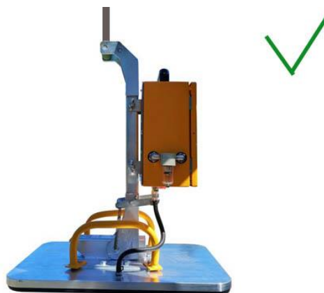
Рисунок 6.3.1 Позиционирование захвата при подъеме груза
